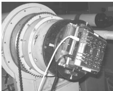
Рис. 1. ПЗЗ-камера Arophee Alta U47 встановлена на МАК в 2010 р.
