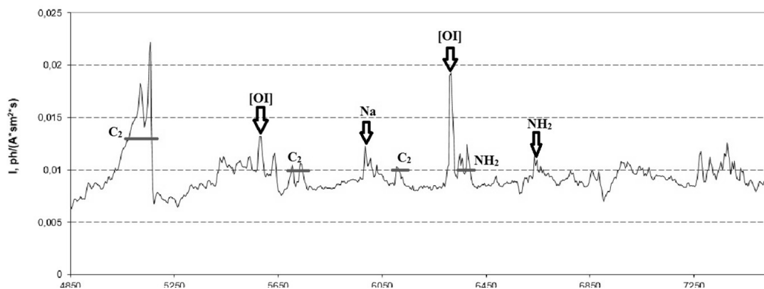
Рис. 1. Емісії в спектрі комети 8P/Tuttle
