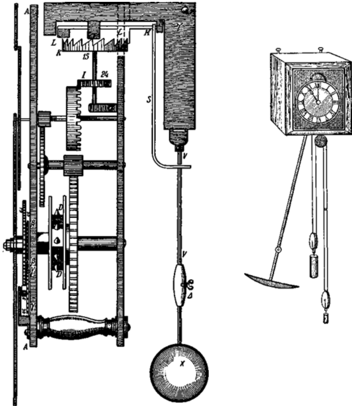
Рис. 2. Годинник з маятником
