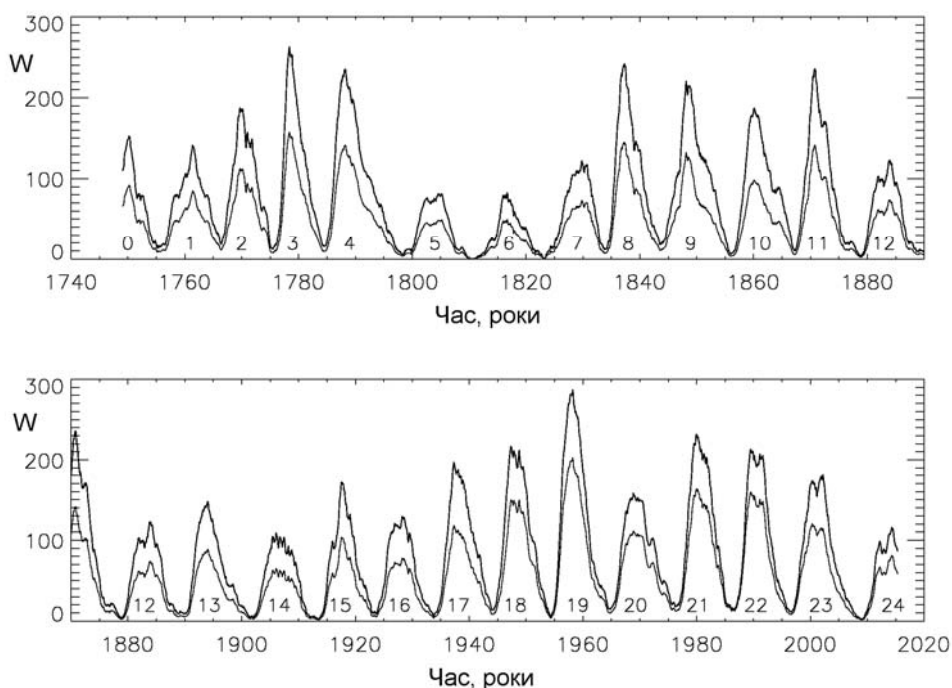
Рис. 1. Зміна з часом місячного згладженого відносного числа сонячних плям W. Товща лінія, що лежить вище, характеризує ревізований ряд. Вказані номери циклів сонячної активності.
