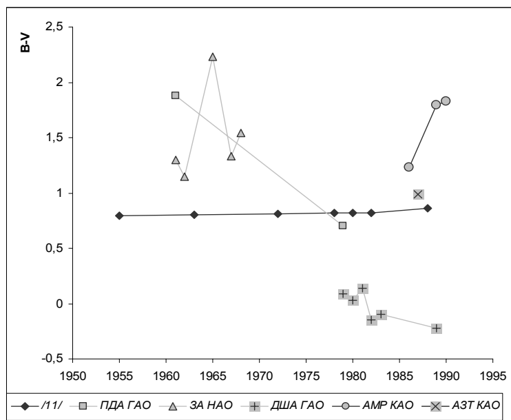
Рис. 4. Значення показників кольору B(T)-V_{\text{eph}} , отриманих за цифровими зображеннями фотоплатівок у порівнянні з опублікованими в роботі [3]
