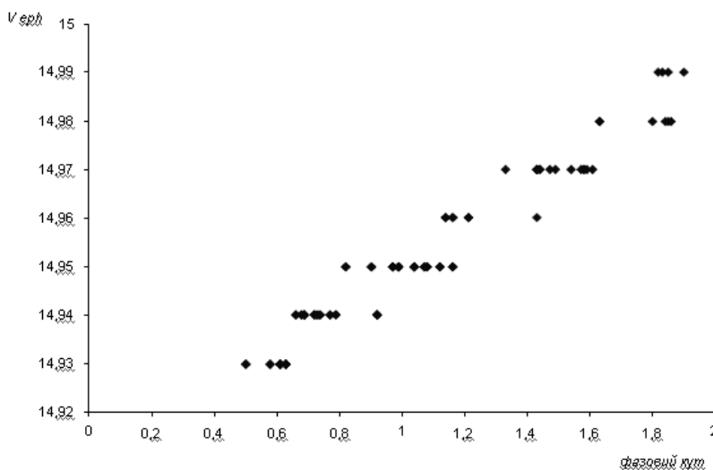
Рис. 2. Розподіл по фазових кутах ефемеридних значень M_{\text{Verh}} , редукованих до середньої опозиції
