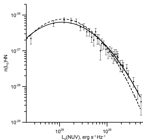
Рис. 3. Те ж, що рис. 1, але для NUV континууму
