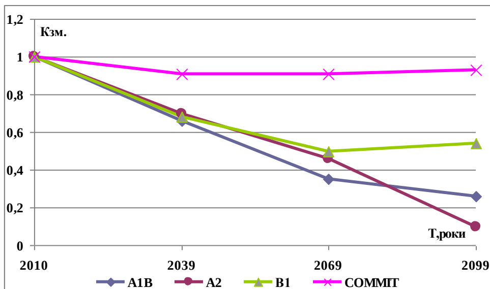
Рис.2. Прогнозні значення коефіцієнтів змін k_{зм} максимального стоку весняного водопілля для середньої (Подільської) та нижньої (Причорноморської) частин басейну р.Дністер за моделлю NCAR_CCSM3 (сценарії A1B, A2,B1, COMMIT)
