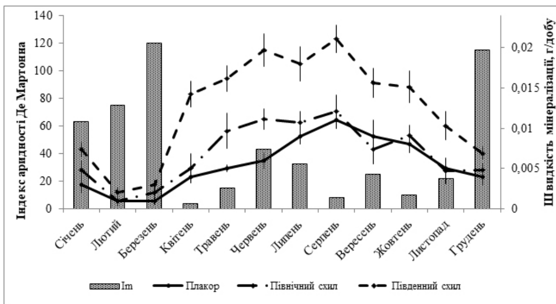
Рис. 1. Динаміка швидкості мінералізації целюлози у лісовій підстилці Голосіївського лісу протягом 2018 року на ділянках з різним типом мікрорельєфу у порівнянні з індексом аридності Де Мартонна.
