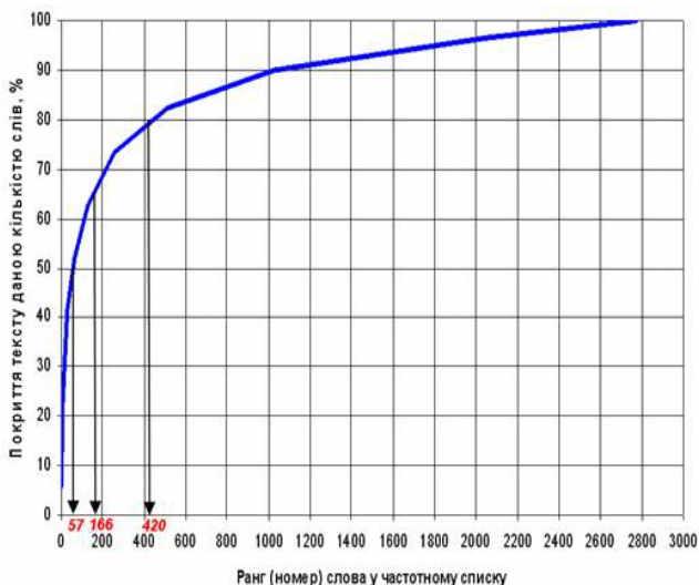
Рис. 3. Діаграма покриття тексту Е. Хемінгуей частотним списком у 2,7 тис. слів. Числа N_{50\%}=57 , N_{66,7\%}=166 , N_{80\%}=420
