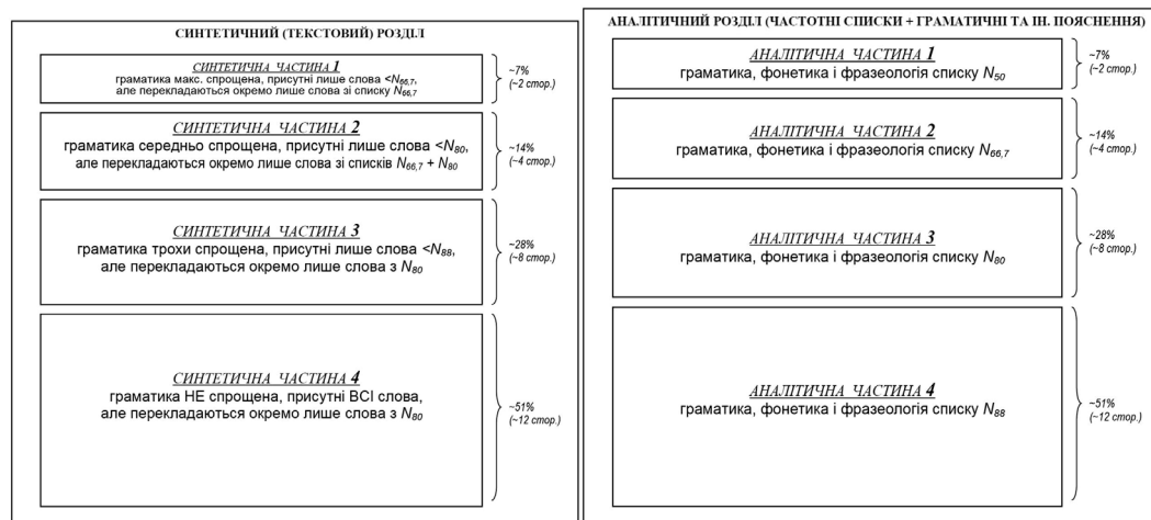
Рис. 5. Схема розбивки синтетичної та аналітичної частин на базі тексту Е. Хемінгуей
