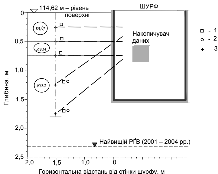
Рис. 1. Станція "Шурф" для спостереження за зоною аерації з вказаним ґрунтовим профілем, що моделюється: 1 – датчик вологості ML2x; 2 – датчик тиску SWТ6; 3 – точки встановлення датчиків (на схемі шурфу); т/г – техногенний шар ґрунту; гум – гумусований шар ґрунту; еол – шар корінного ґрунту (пісок еолового генезису)
