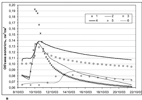
с. 4. Порівняння режиму природної вологості та розрахованої в результаті моделювання для обраних періодів: 1 – натурні дані, глибина 0,25 м; 2 – "модельні" дані; 3 – натурні дані, глибина 0,5 м; 4 – "модельні" дані; 5 – натурні дані, глибина 1,25 м; 6 – "модельні" дані
