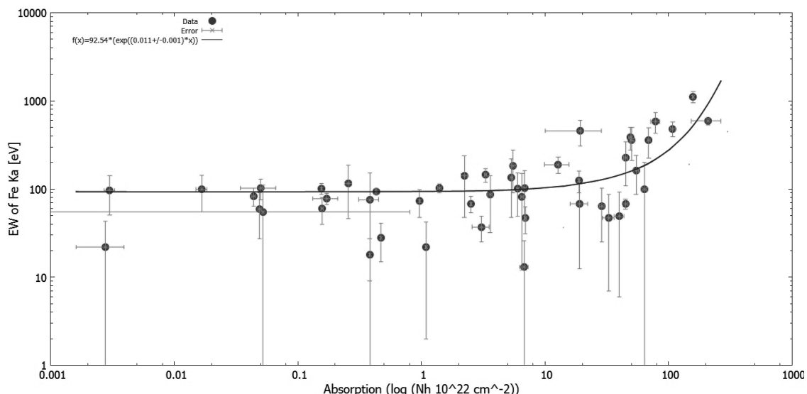
Рис. 2. Еквівалентна ширина лінії Fe K \alpha як функція від величини стовпчикового поглинання
