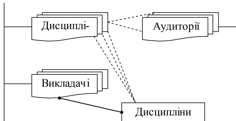
Рисунок 4.3 – Мережний спосіб організації даних
