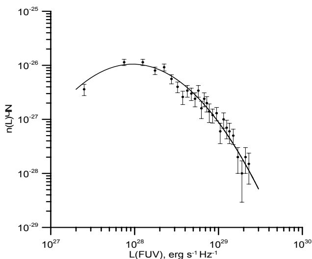
Рис. 2. Функція світності вибірки LCGs галактик, отримана за їх випромінюванням у далекому УФ континуумі та апроксимована log-нормальним розподілом з параметрами L_0 = 0.946 \times 10^{28} \text{ ерг} \cdot \text{с}^{-1} \cdot \text{Гц}^{-1} , L_1 = 2.910 \times 10^{28} \text{ ерг} \cdot \text{с}^{-1} \cdot \text{Гц}^{-1} та a = 0.445 , які визначено за допомогою ММП
