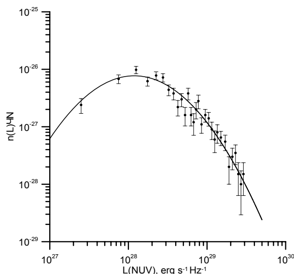
Рис. 3. Функція світності вибірки LCGs галактик, отримана за їх випромінюванням у близькому УФ континуумі та апроксимована log-нормальним розподілом з параметрами L_0 = 1.186 \times 10^{28} \text{ ерг} \cdot \text{с}^{-1} \cdot \text{Гц}^{-1} , L_1 = 3.988 \times 10^{28} \text{ ерг} \cdot \text{с}^{-1} \cdot \text{Гц}^{-1} та a = 0.412 , які визначено за допомогою ММП
