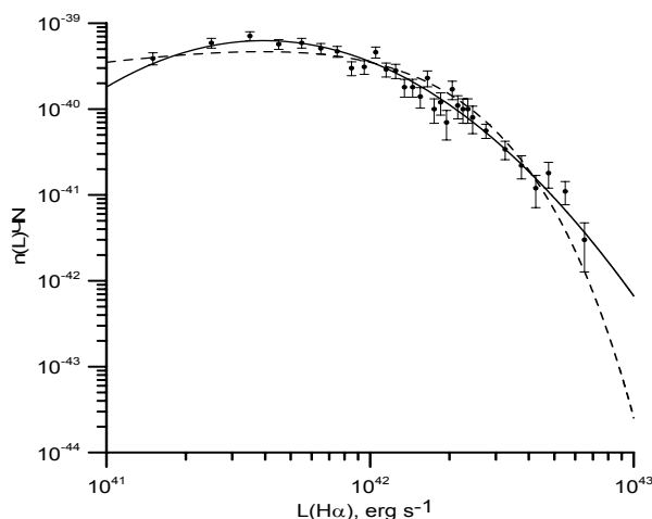
Рис. 1. Функція світності вибірки LCGs галактик, отримана за їх випромінюванням у емісійній лінії H \alpha областей іонізованого водню HII та апроксимована log-нормальним розподілом з параметрами L_0 = 3.96 \times 10^{41} \text{ ерг} \cdot \text{с}^{-1} , L_1 = 8.5 \times 10^{41} \text{ ерг} \cdot \text{с}^{-1} та a = 0.657 , які визначено за допомогою ММП (суцільна лінія). Апроксимація ФС вибірки LCGs галактик функцією Шехтера – пунктирна лінія.
