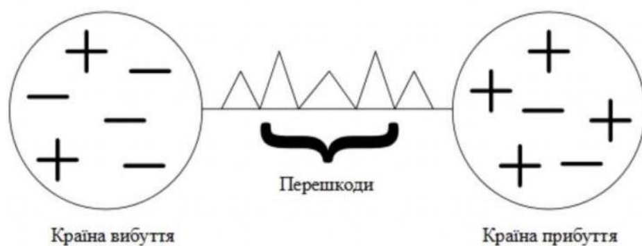
Рис. 1. Схема моделі притягання – відштовхування.
