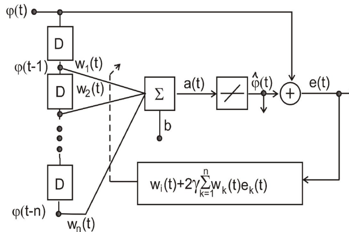
Рис. 2. Нейромережа прогнозу стоку р. Дністер
