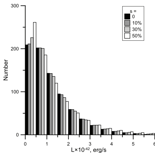
Рис. 3. Функції світності для згенерованого імітаційного каталогу (18) та усереднена функція світності для згенерованого імітаційного каталогу з "шумом" (21), який задається різним рівнем величини максимальної відносної похибки s . Значення s та відповідний колір колонок приведено на рисунку
